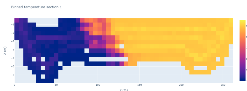
Représentation du mélange de température à la confluence Rhône-Saône
