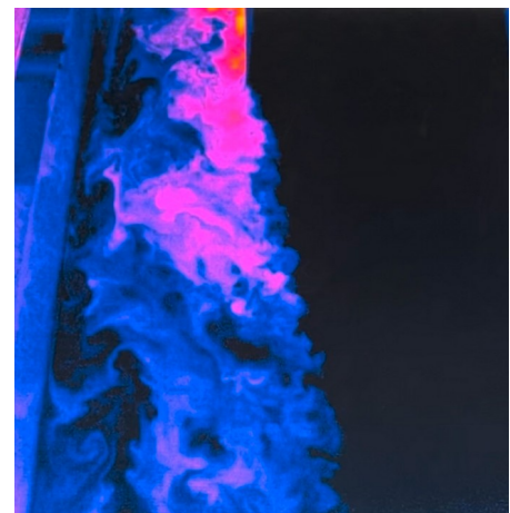
Visualisation du mélange en canal avec une caméra thermique
